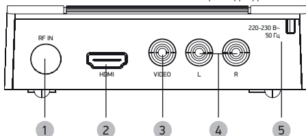
Общий вид задней панели
